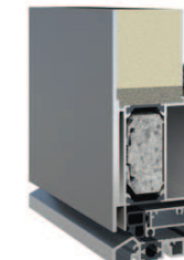
Wärmeschutzfüllung 60 mm in Ausführung: Flügelüberdeckend
